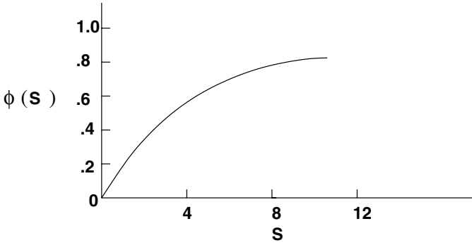
Figure 3.8. Kussner function.
